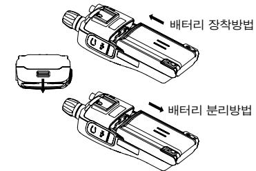
그림5-2) 배터리 장착 및 분리방법
