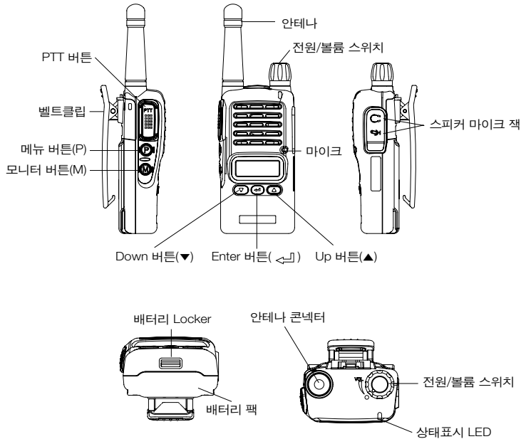
그림3-1) XQ Series 외형 및 주요기능
