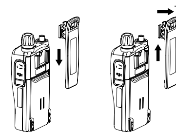
그림5-3) 벨트클립 장착 및 분리방법
